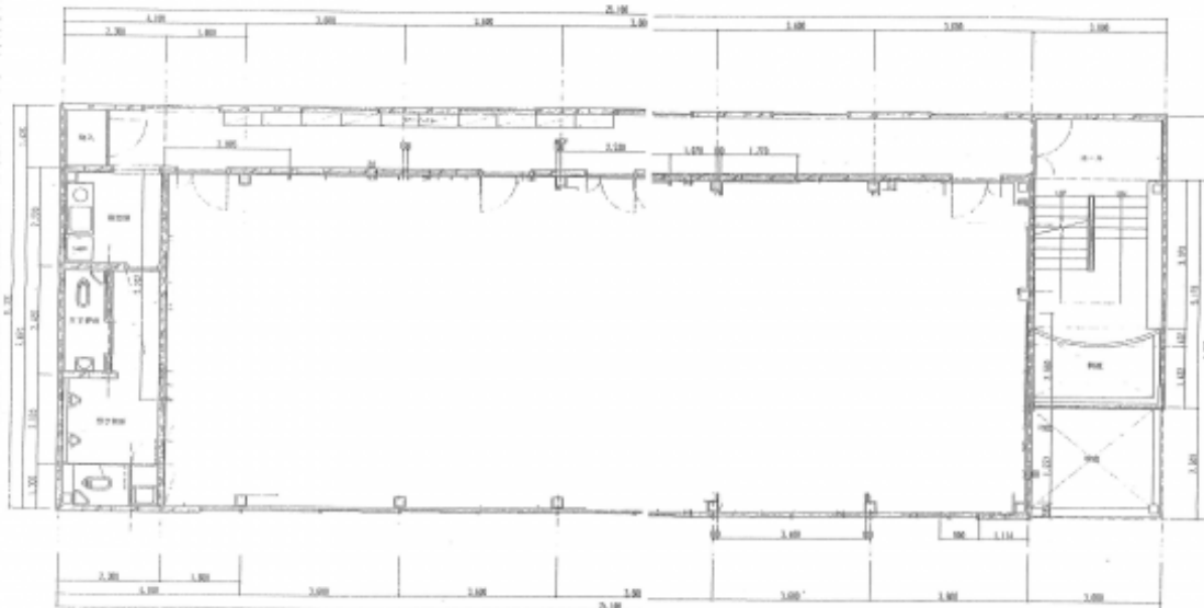
松山第一ビル 2F 平面図 S=1/50
